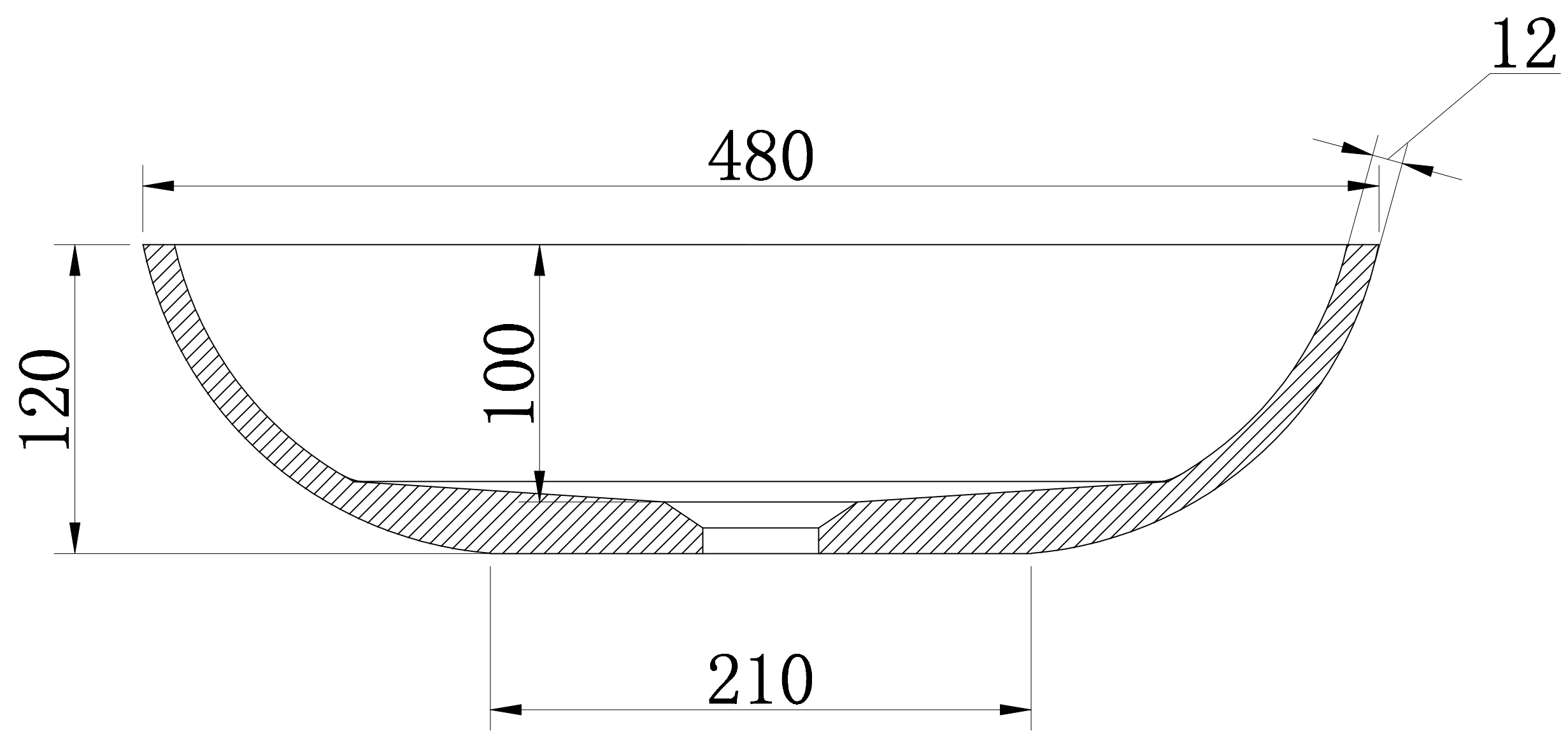
A-A
