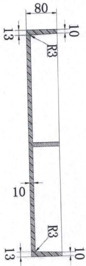
A-A
