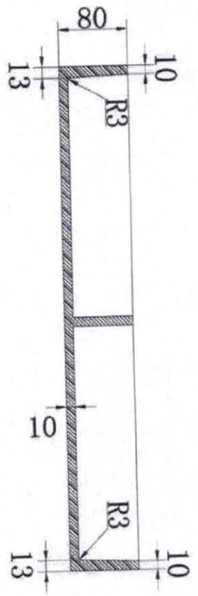
A-A
